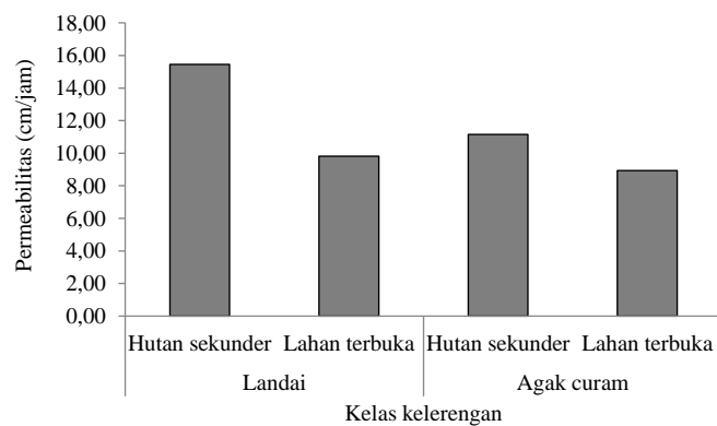
Gambar 5. Permeabilitas Tanah pada Kelas Kelerengan Berbeda.
