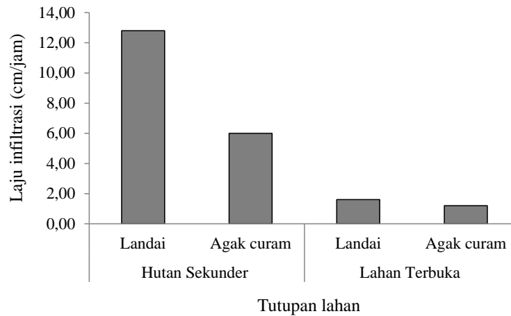
Gambar 2. Laju Infiltrasi pada Tutupan Lahan Berbeda.
