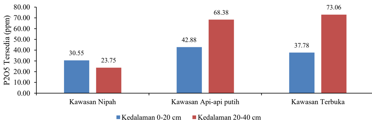
Gambar 7. Diagram P 2 O 5 Tersedia Tanah pada Kawasan Nipah, Api-api Putih, dan Terbuka di Kedalaman 0-20 cm dan 20-40 cm.
