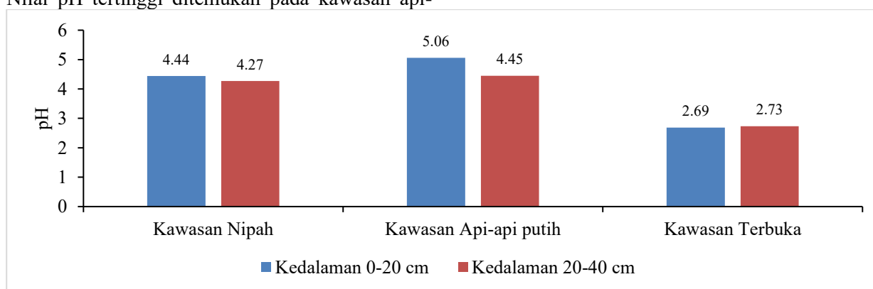
Gambar 6. Diagram pH Tanah pada Kawasan Nipah, Api-api Putih, dan Terbuka di Kedalaman 0-20 cm dan 20-40 cm
