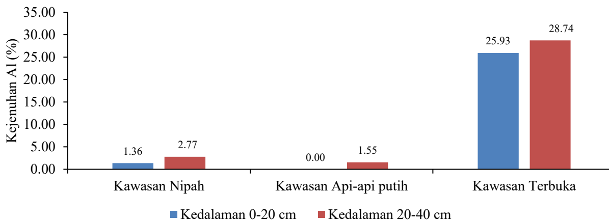
Gambar 4. Diagram Kejenuhan Aluminium (Al) Tanah pada Kawasan Nipah, Api-api Putih, dan Terbuka di Kedalaman 0-20 cm dan 20-40 cm.
