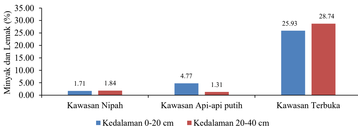
Gambar 12. Diagram Minyak dan Lemak Tanah pada Kawasan Nipah, Api-api Putih, dan Terbuka di Kedalaman 0-20 cm dan 20-40 cm
