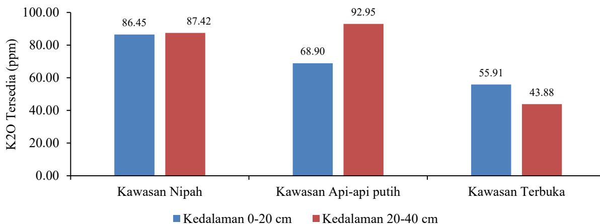
Gambar 8. Diagram K 2 O Tersedia Tanah pada Kawasan Nipah, Api-api Putih, dan Terbuka di Kedalaman 0-20 cm dan 20-40 cm.
