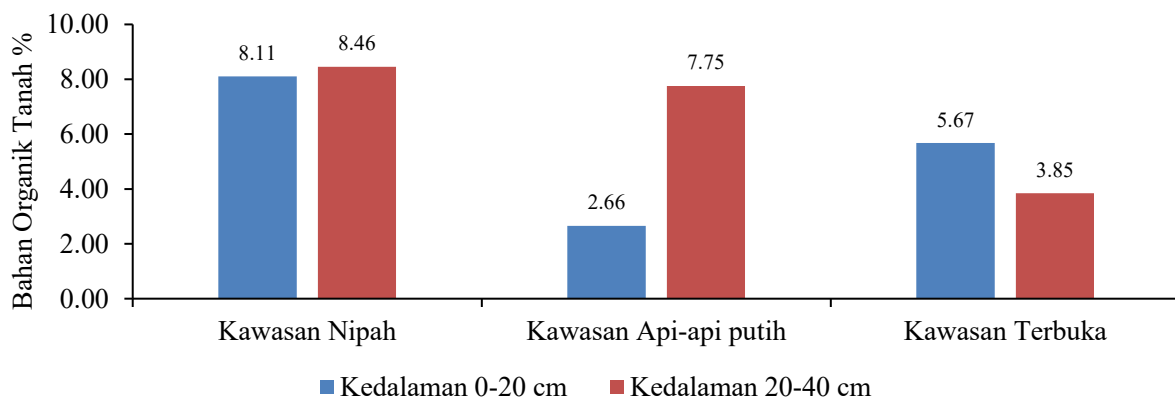
Gambar 2. Diagram Bahan Organik Tanah pada Kawasan Nipah, Api-api Putih, dan Terbuka di Kedalaman 0-20 cm dan 20-40 cm.
