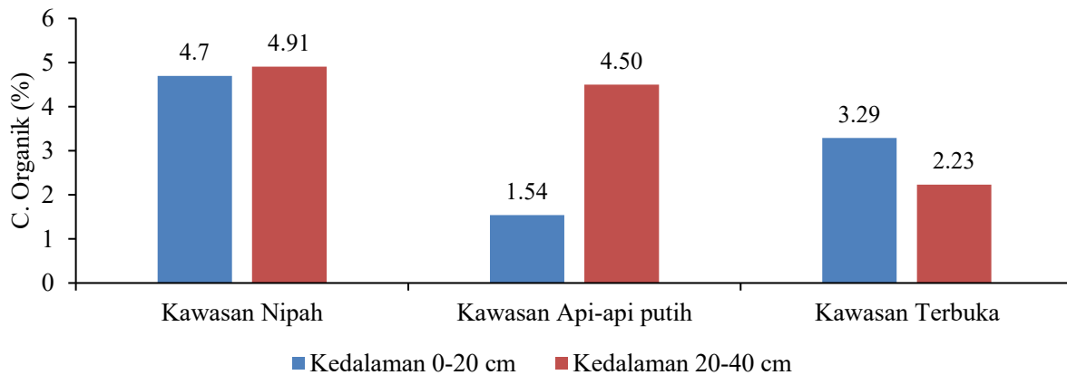
Gambar 9. Diagram C-Organik Tanah pada Kawasan Nipah, Api-api Putih, dan Terbuka di Kedalaman 0-20 cm dan 20-40 cm
