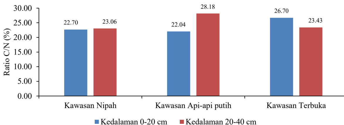
Gambar 11. Diagram Ratio C/N Tanah pada Kawasan Nipah, Api-api Putih, dan Terbuka di Kedalaman 0-20 cm dan 20-40 cm.
