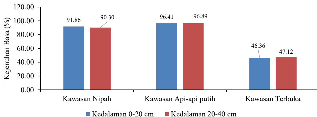
Gambar 3. Diagram Kejenuhan Basa Tanah pada Kawasan Nipah, Api-api Putih, dan Terbuka di Kedalaman 0-20 cm dan 20-40 cm.
