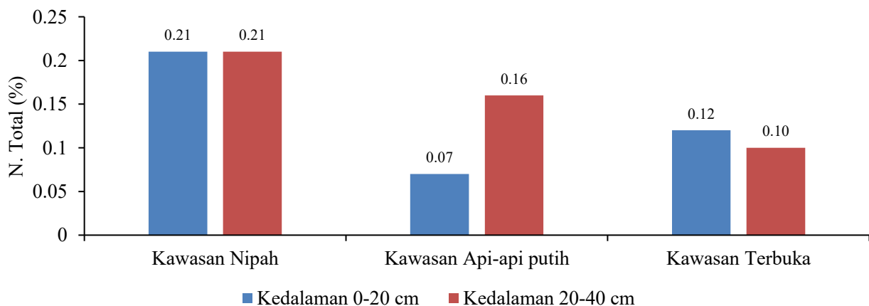
Gambar 10. Diagram N.Total Tanah pada Kawasan Nipah, Api-api Putih, dan Terbuka di Kedalaman 0-20 cm dan 20-40 cm
