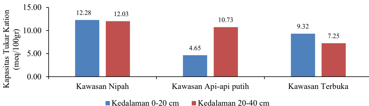
Gambar 5. Diagram Kapasitas tukar Kation Tanah pada Kawasan Nipah, Api-api Putih, dan Terbuka di Kedalaman 0-20 cm dan 20-40 cm.
