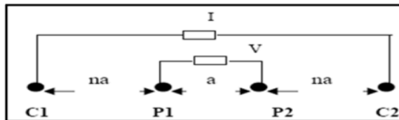
Gambar 1. Susunan Elektroda Konfigurasi Wenner - Schlumberger
