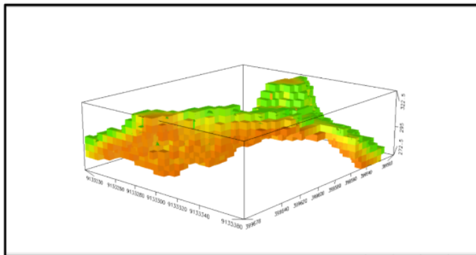
Gambar 8. Hasil Pemodelan 3D Andesit Lapuk
