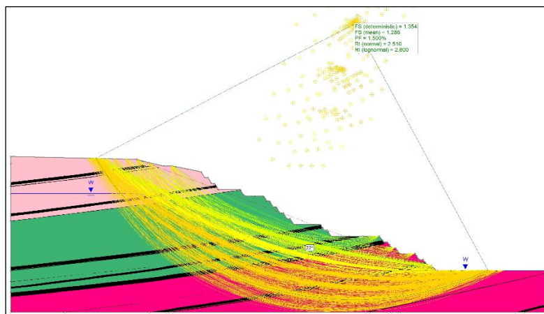
Gambar 9. Hasil Redesain dengan sudut 22° (Olahan Penulis, 2025)
