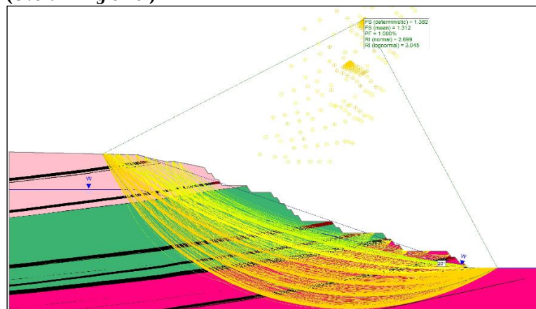
Gambar 10. Hasil Redesain dengan sudut 20° (Olahan Penulis, 2025)
