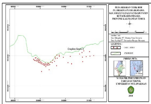
Gambar 3. Sebaran Data Bor
