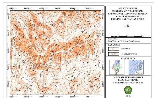
Gambar 1. Topografi Daerah Penelitian
