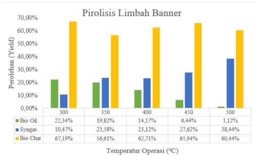
Gambar 3. Grafik Perolehan Produk Pirolisis Limbah Banner
