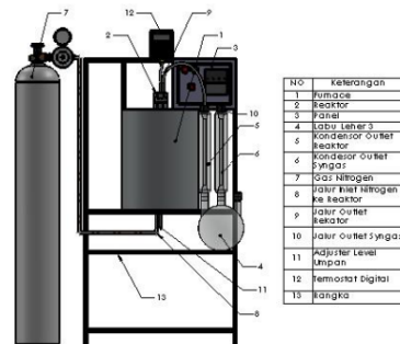
Gambar 1. Rangkaian Alat Pirolisis
