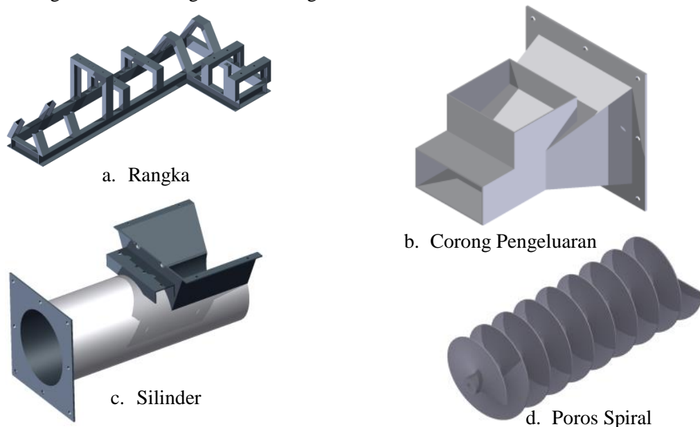
Gambar 1. Komponen Mesin Pencetak Batu Bata
