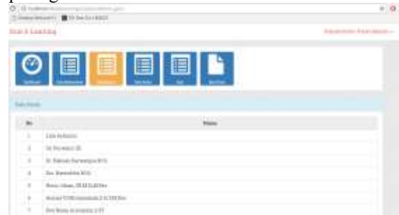
Gambar 3.4 Data Dosen
