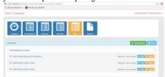
Gambar 3.6 Data Soal
